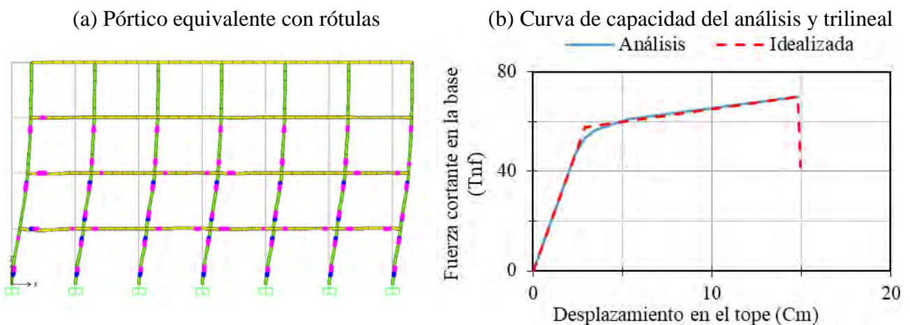
Figura 9.11 Modelo de pórtico equivalente con plasticidad concentrada y curvas de capacidad.
