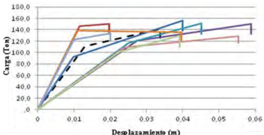
Curvas de capacidad obtenidas para los ocho casos de análisis. Figura 13.15
