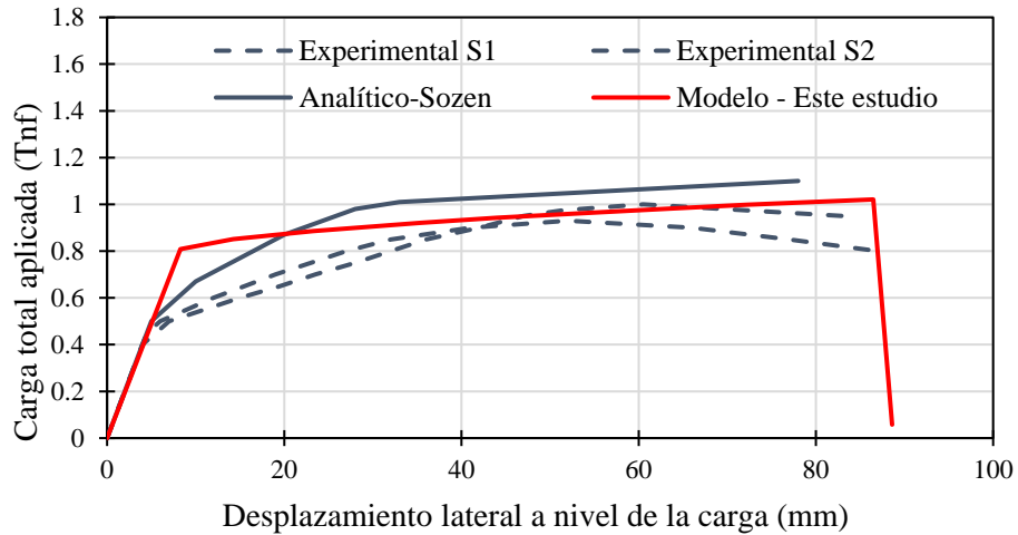
Figura 9.10 Comparación de la curva de capacidad del modelo y de los resultados experimentales.
