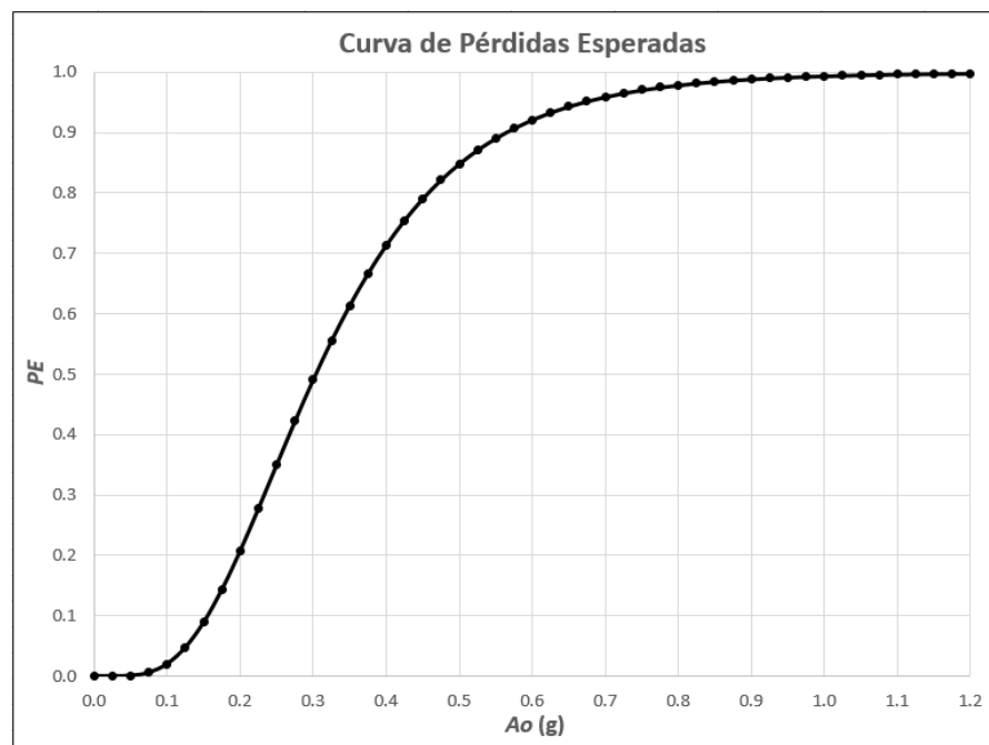
Figura 14.23 Curva de pérdidas esperadas del Conjunto Los Mangos, Puente Plaza Venezuela-Estadios (21A).
