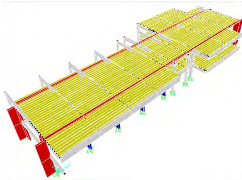
Propuesta conceptual de reforzamiento para la Estación de El Valle.
