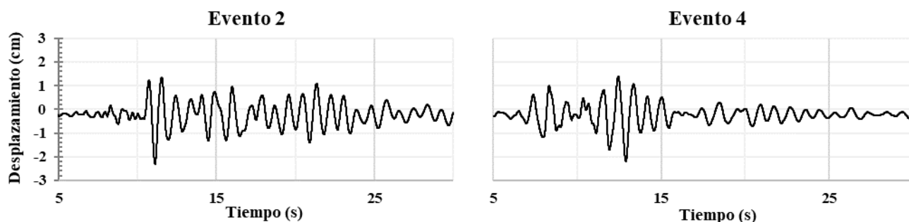
Historia del desplazamiento en el último nivel, dirección longitudinal (L) del edificio para los eventos sísmicos 2 y 4.
