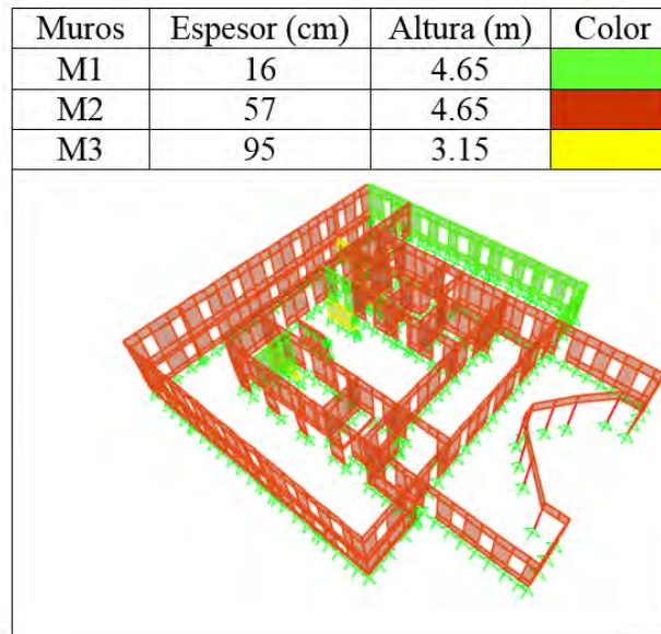
Figura 11.15 Características y distribución de los muros del modelo de la Villa "Santa Inés"
