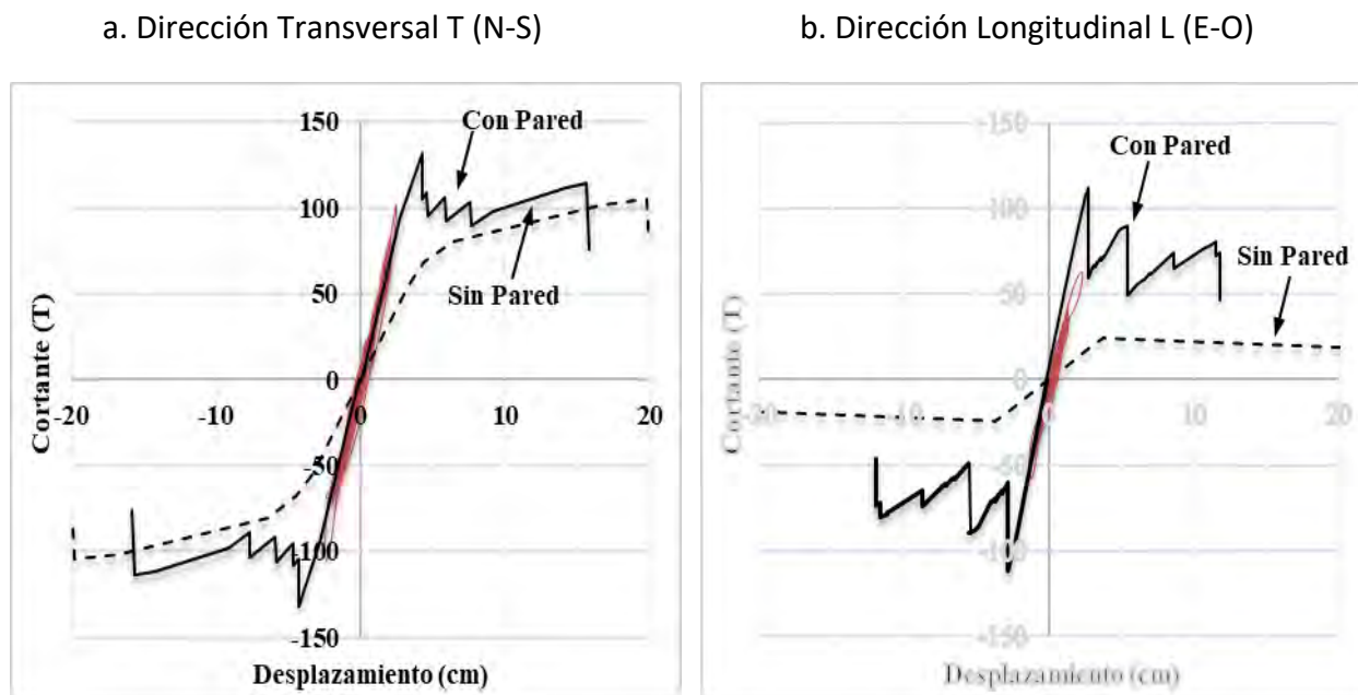
Curva de capacidad (AENL) de pórticos representativos del edificio (negro). Respuesta dinámica (ADNL) (naranja) para el Evento 2, y curva de capacidad del pórtico sin paredes. Sismo 1967.
