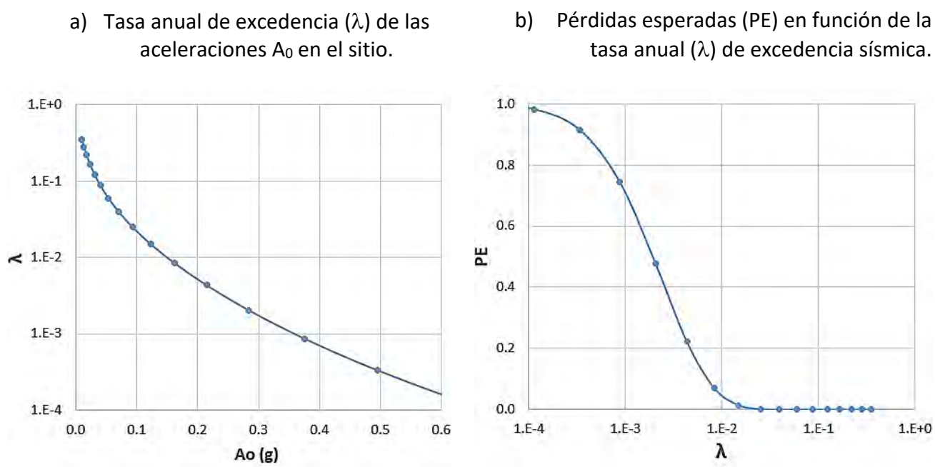
Curva de amenaza sísmica en el sitio y pérdidas esperadas en función de la tasa anual de excedencia sísmica ( \lambda ). Tramo 20 del Puente Tramo Elevado UCV.
