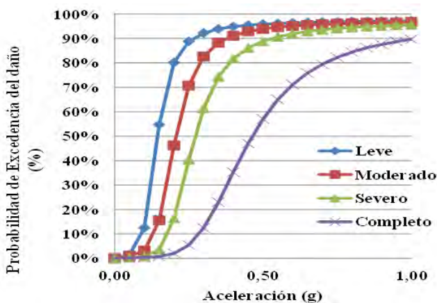
Curvas de fragilidad para Roca (Mz R3-To). El cuadro indica los valores de aceleración para 50% de probabilidad de excedencia. Figura 13.16
