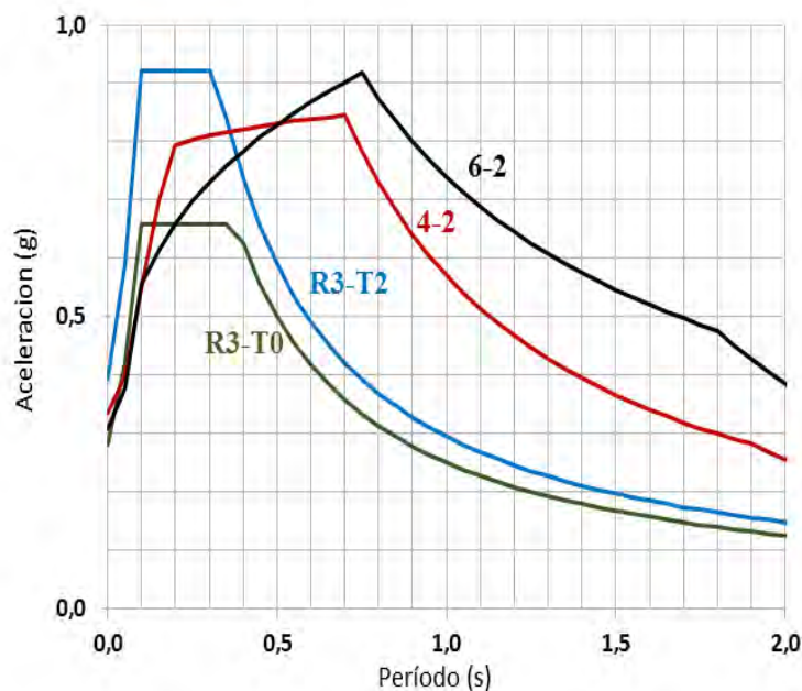
Espectros de aceleraciones para cuatro condiciones de sitio. Figura 5.7
