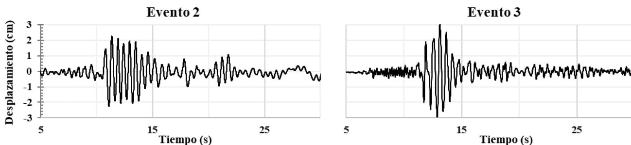
Historia del desplazamiento en el último nivel, dirección transversal (T) del edificio para los eventos sísmicos 2 y 3.
