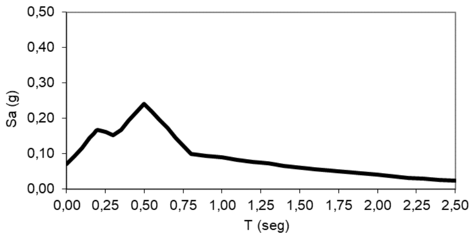
Espectro en LPG, adaptado de Alonso (1975)
